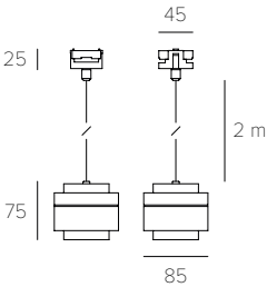
Adjustable cable. Cavo regolabile.
